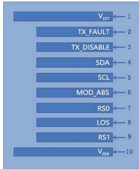
底部视图
