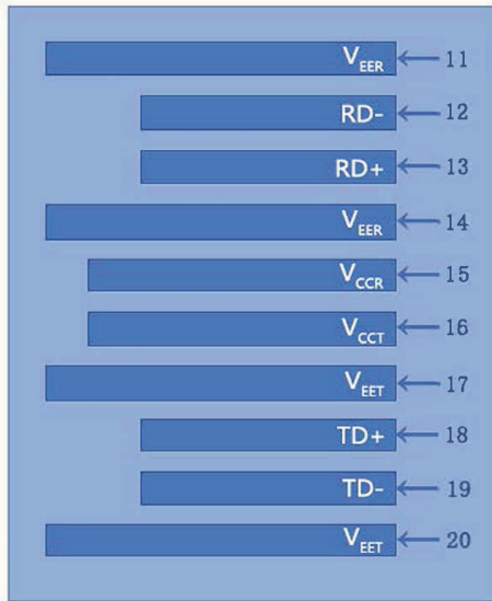
顶部视图
