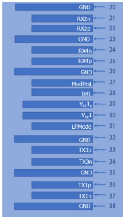
顶部直视图
