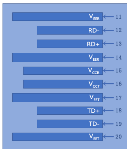
顶部直视图
