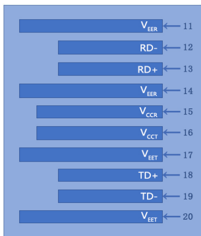
顶部视图
