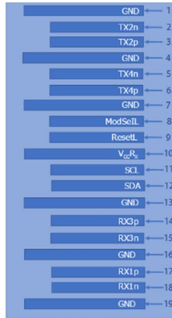
底部直视图
